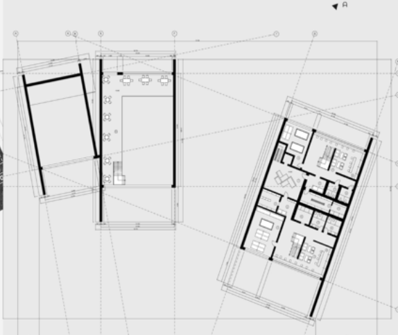
Рис. 4. Проект рекреаційно-оздоровчого комплексу в с. Стара Гута Івано-Франківської обл.
