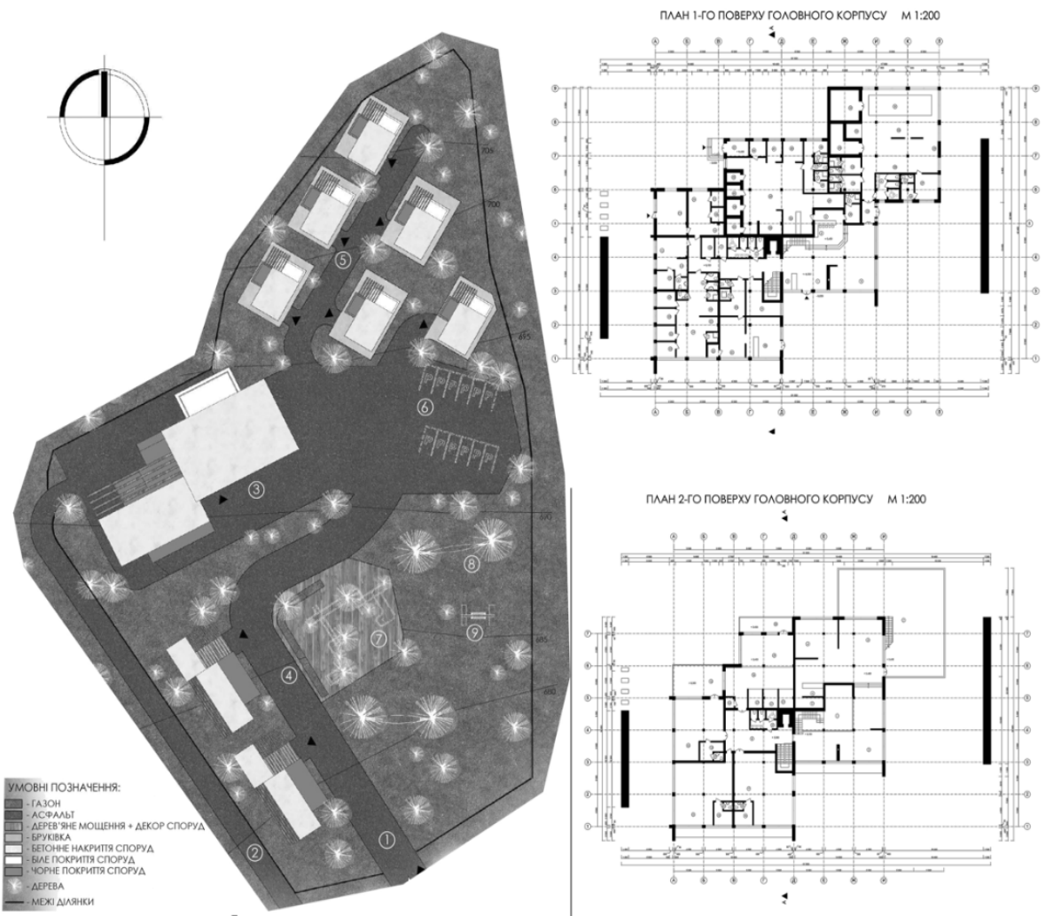
Рис. 3. Проект гірського рекреаційного комплексу в с. Стара Гута Івано-Франківської обл.
