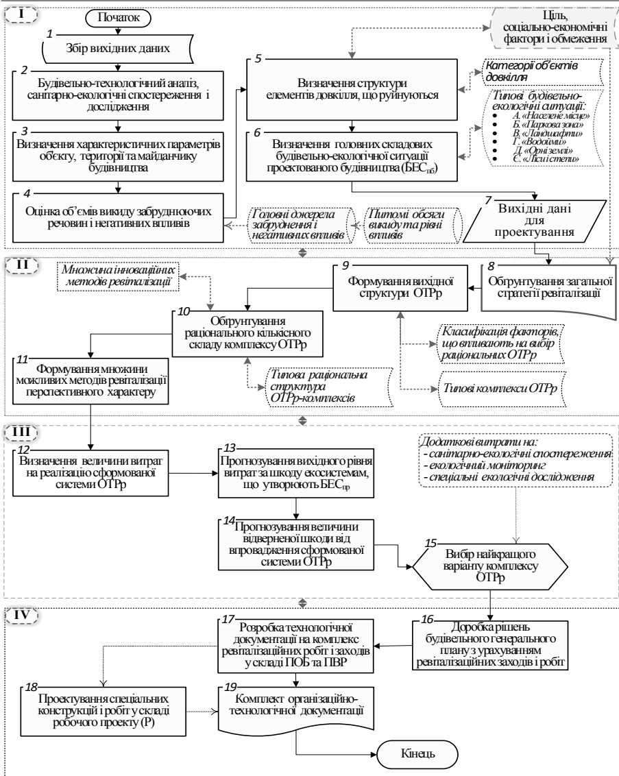
Рис. 1. Схема методики проєктування організаційно-технологічних рішень ревіталізації процесів будівельного виробництва:
