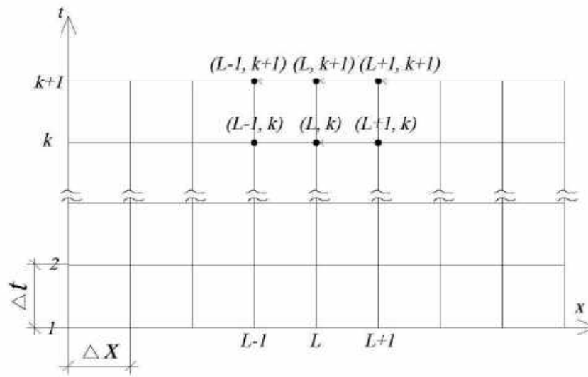
Рис.1. Різницева схема.
